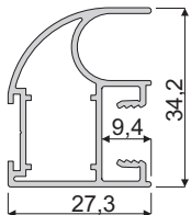
Profil TOKYO 2
